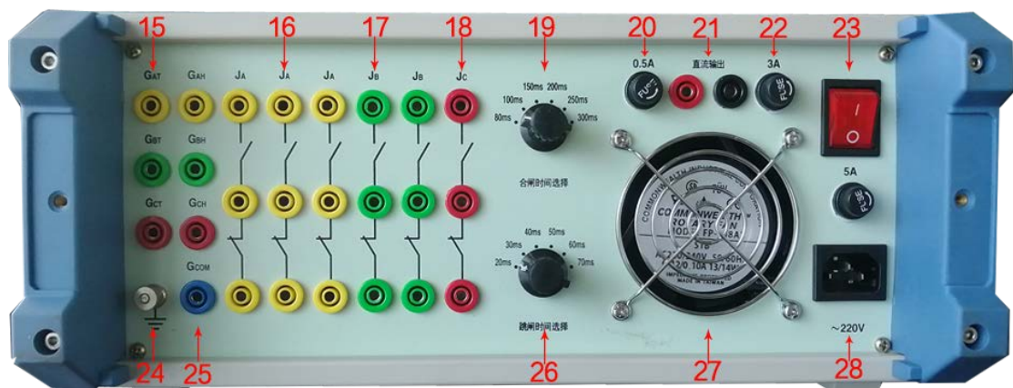
图-2 MDL-A 仪器背板功能
